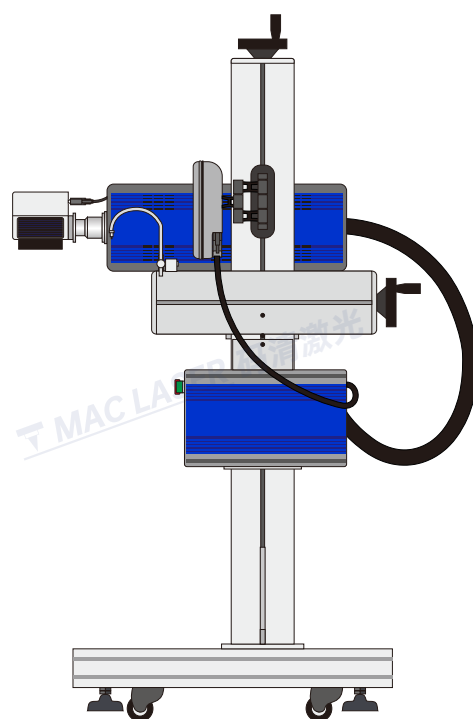
设备左侧
