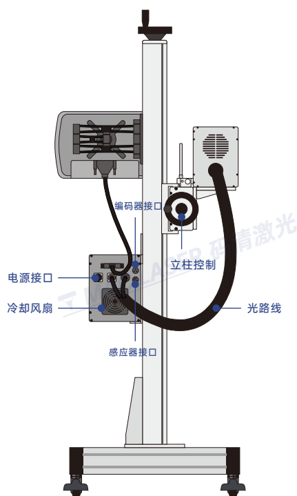
设备背面
